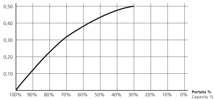
Curve forza / carico - Traferro (su acciaio comune) Diagram WLL / air gap
