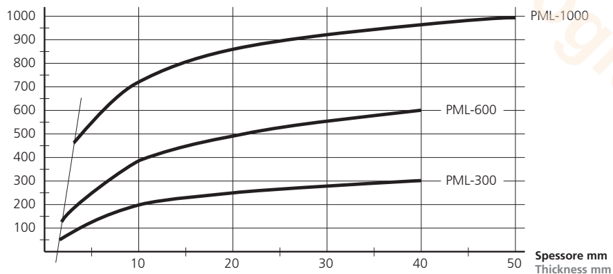
Curve forza / carico - Traferro (su acciaio comune) Diagram WLL / air gap
